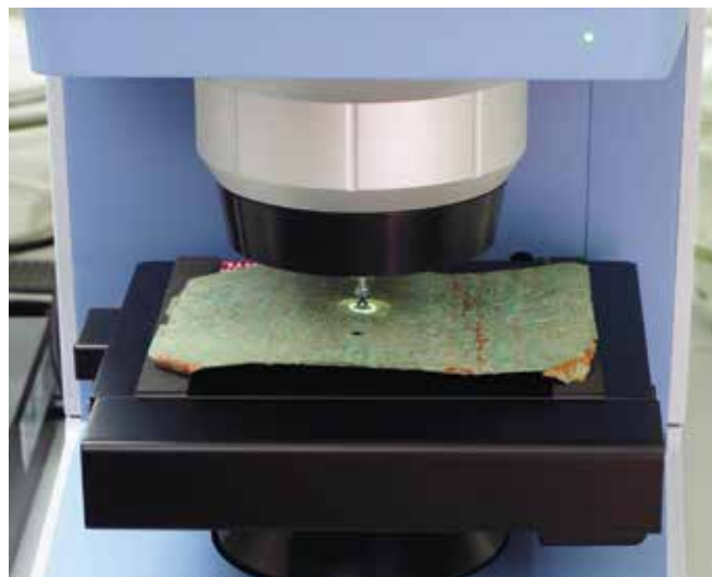
Modernes Infrarotspektrometer-Mikroskop („FTIR-ATR-Mikroskop“, ATR = Attenuated Total Reflection). Kleinere Objekte mit bis zu mehreren Zentimetern Höhe, wie die hier auf dem Objektisch liegende, kupferne Schrifttafel, können ohne Probenahme untersucht werden. Bei der FTIR-ATR-Messung (rechts) senkt sich der motorisch gesteuerte ATR-Sensorstift auf die Probe herab und berührt diese mit seinem konisch zulaufenden Ende über eine Kreisfläche von nur 0,1 mm Durchmesser. Die in die Germaniumspitze eingelenkte Infrarotstrahlung wird am Messfenster reflektiert, nimmt dabei die Information von der unmittelbar benachbarten Probe auf und bewegt sich weiter zum Detektor, der das Bild des Spektrums erzeugt. (Fotos: BLfD, Martin Mach)
