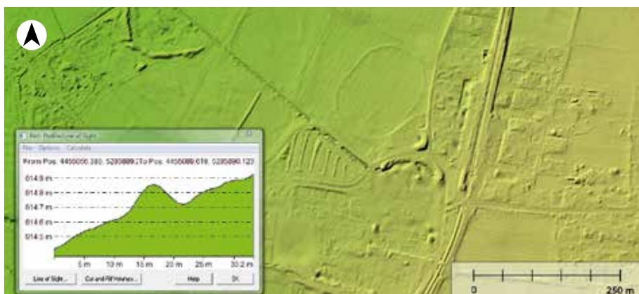
Benediktbeuern. Digitales Geländemodell der Remonten-Laufbahn mit gemessenem Querprofil. DGM-Rasterweite 1 m, Aufsicht (Geodaten: Landesamt für Digitalisierung, Breitband und Vermessung München; Bearbeitung: Hermann Kerscher)
