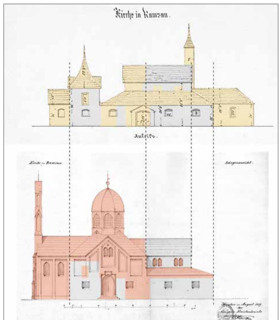
Ramsau, Pfarrkirche Maria Loreto, Baualtersplan. Oben Aufmaß des Vorgängerbaus von 1628/1639 vor der Umgestaltung, darunter Planung zum Umbau 1859, Ansichten von Süden. Grau: vom Vorgängerbau übernommenen Substanz, Gelb: abgetragene Bauteile, Rot: neu errichtete Bauteile (Pläne: Archiv Staatliches Bauamt Rosenheim / Barthel & Maus)
