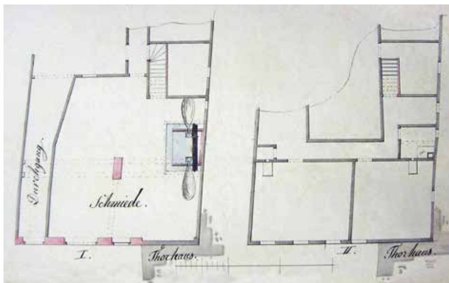
Bamberg, Untere Königstr. 37, Erd- und Obergeschossgrundriss des Vorderhauses zur Versteinerung des südlichen Teils der Fassade, erstellt 1847 von Maurermeister Joseph Dennefeld (Plan: Städtische Aktenregistratur Bamberg)
