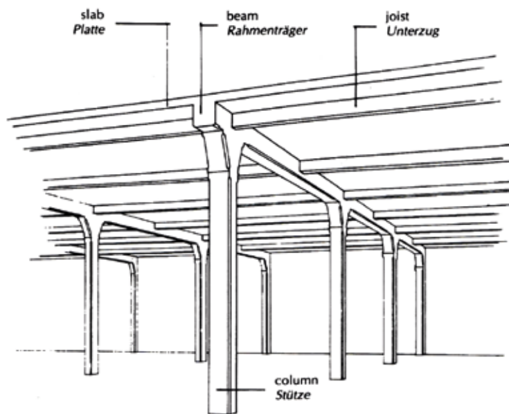
Schematische Darstellung eines Hennebique-Rahmentragwerk, 1904 (aus: Beton-Atlas, München-Düsseldorf 1995)
