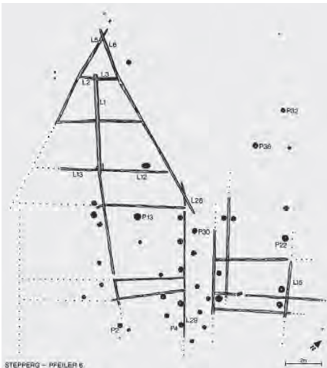
Grundrissplan Pfeiler 6 (Zeichnung: Marcus Prell/BGfU, 1993)
